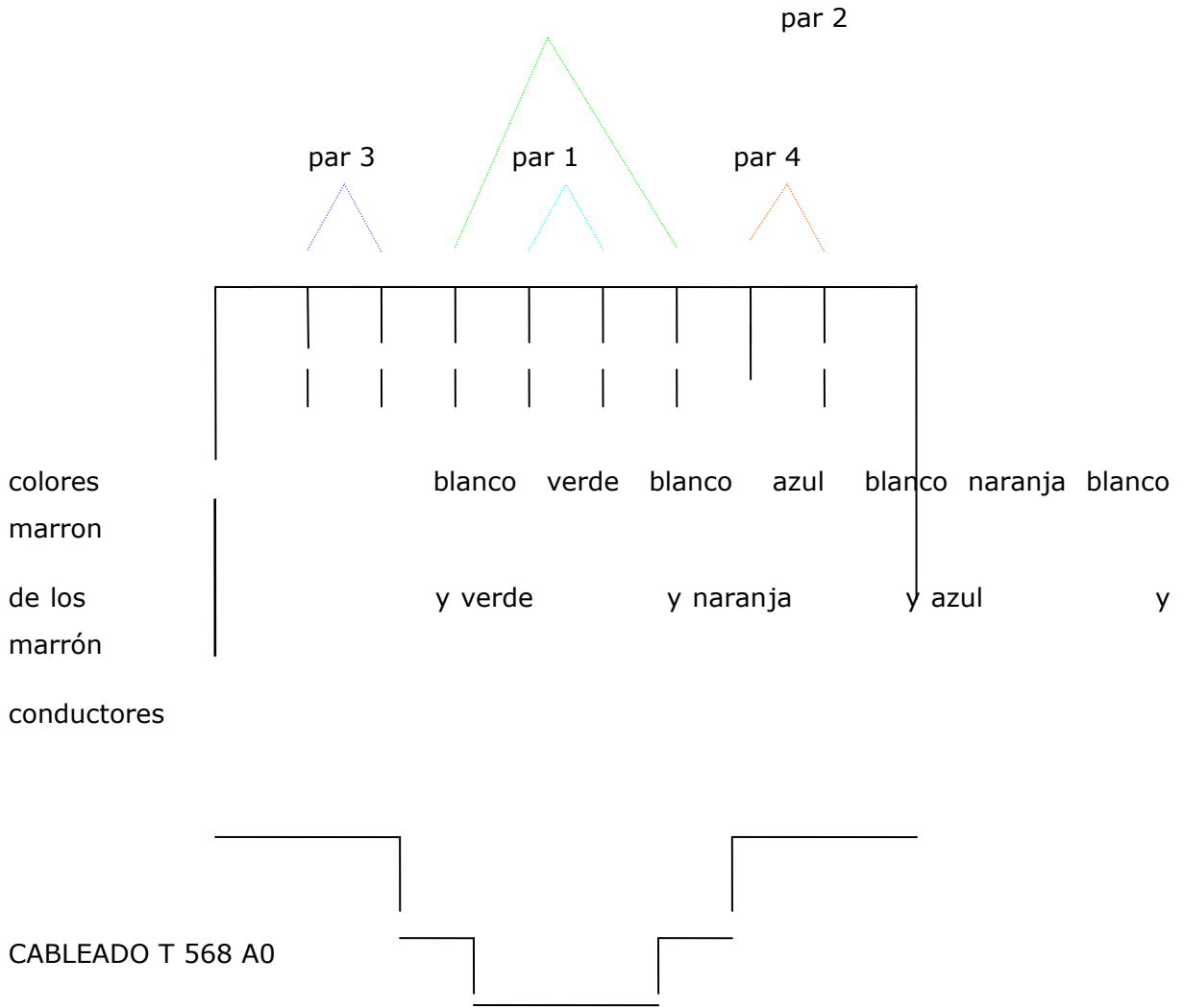
Conector modular de 8 posiciones (vista frontal)
